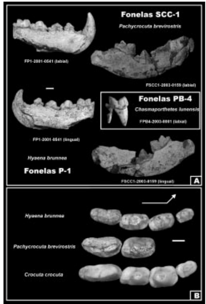
Fig. 2. Hiénidos registrados en los nuevos yacimientos paleontológicos de Fonelas. A , Elementos de la dentición inferior de Hyaena brunnea (fragmento de hemimandíbula derecha; Fonelas P-1), Pachycrocuta brevirostris (fragmento de hemimandíbula derecha; Fonelas SCC-1) y Chasmaporthetes lunensis (M1, derecho; Fonelas PB-4). B , Comparativa, en vista oclusal, de la dentición inferior de Hyaena brunnea (Fonelas P-1) y Pachycrocuta brevirostris (Fonelas SCC-1) en relación con Crocuta crocuta intermedia del yacimiento mesopleistoceno de Villacastín (Segovia). Escalas gráficas: 1 cm Fig. 2. Hyaenids from the new paleontological sites at Fonelas. A , Lower dentition of Hyaena brunnea (right hemimandible fragment; Fonelas P-1), Pachycrocuta brevirostris (right hemimandible fragment; Fonelas SCC-1) and Chasmaporthetes lunensis (right M 1 ; Fonelas PB-4). B , Compared lower dentition in occlusal view of Hyaena brunnea (Fonelas P-1) and Pachycrocuta brevirostris (Fonelas SCC-1) relative to Crocuta crocuta intermedia from the mesopleistocene site of Villacastín (Segovia). Scale bar: 1 cm
