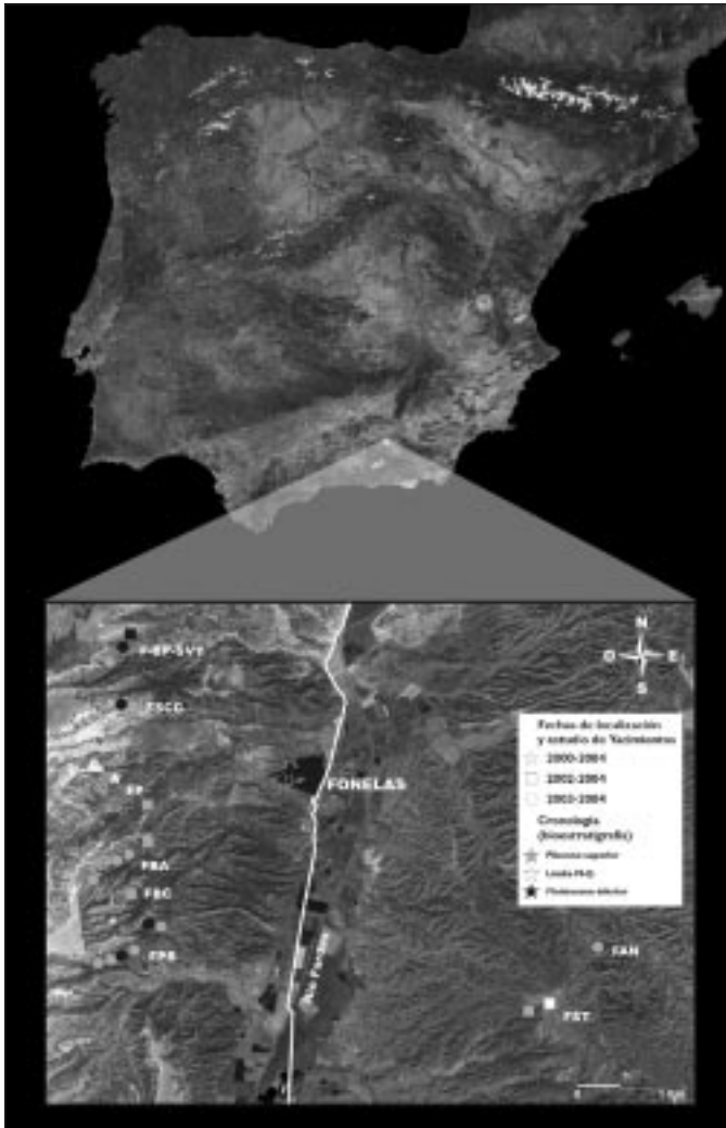
Fig. 1. Localización geográfica de la comarca de Fonelas en la Península Ibérica (imagen satélite de España y Portugal modificada de http://visibleearth.nasa.gov/Countries/Spain/286_2.html ; Jacques Descloitres, MODIS Land Rapid Response Team at NASA/GSFC) y ubicación de los distintos yacimientos identificados en el marco del Proyecto Fonelas en las proximidades de dicho municipio granadino (SIG Proyecto Fonelas, IGME)
