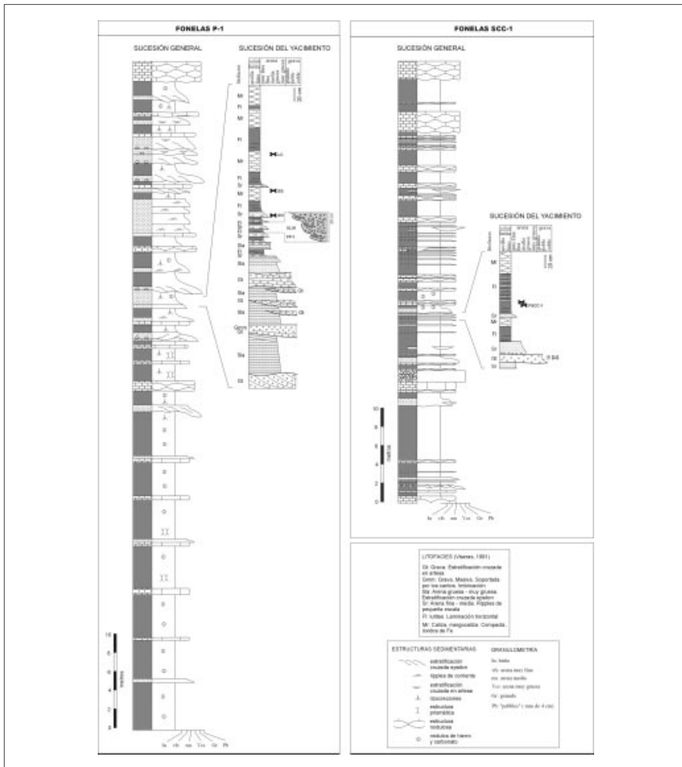
Fig. 4. Sucesiones generales y de detalle de los yacimientos Fonelas P-1 (por Viseras, Soria y Durán) y Fonelas SCC-1 (por Blanco y Bermúdez). En la sucesión de detalle de Fonelas P-1 se han identificado 4 horizontes fosilíferos, procediendo la colección de referencia del horizonte basal, nominado informalmente como ULIA (FP-1)
